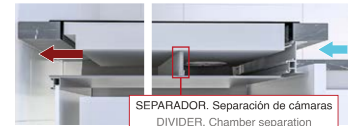
SEPARADOR. Separación de cámaras DIVIDER. Chamber separation
